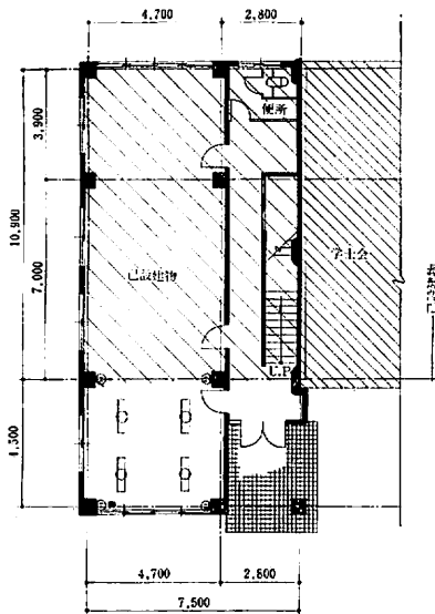
1階平面図
